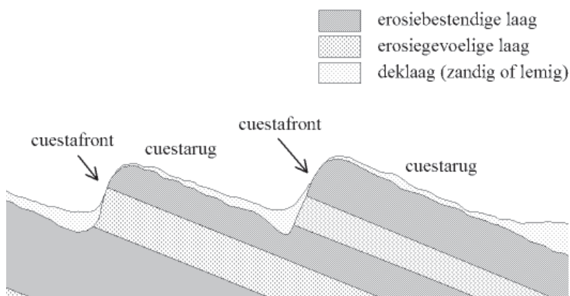
Schematische doorsnede van 2 opeenvolgende cuesta's (Chantal Martens)
